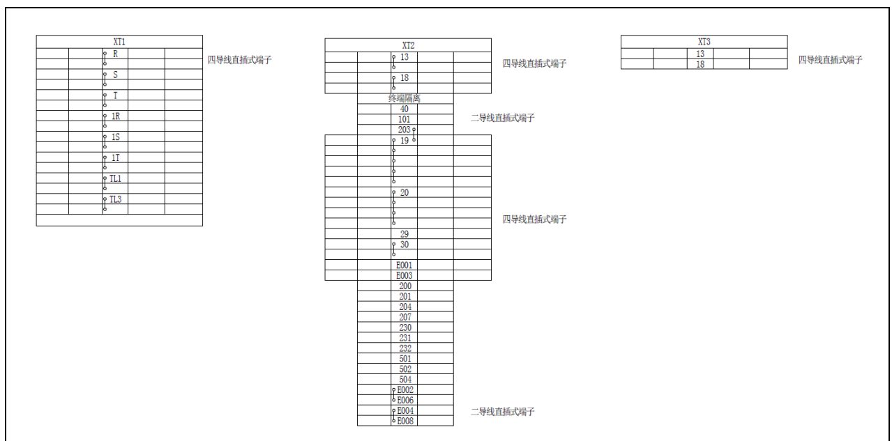
图 11.8 接线端子排接线图（ER50/170/220）
