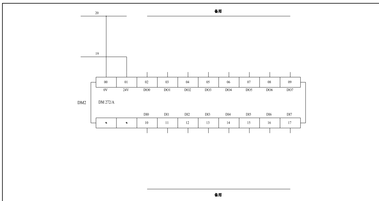
图 11.4 通用输入输出模块接线图
