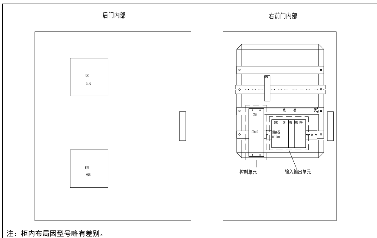
图 1.9 电柜内部布局（3）
