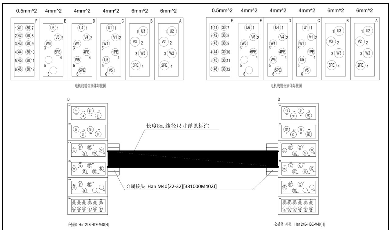
图 11.14 动力航插接线图 (ER500)
