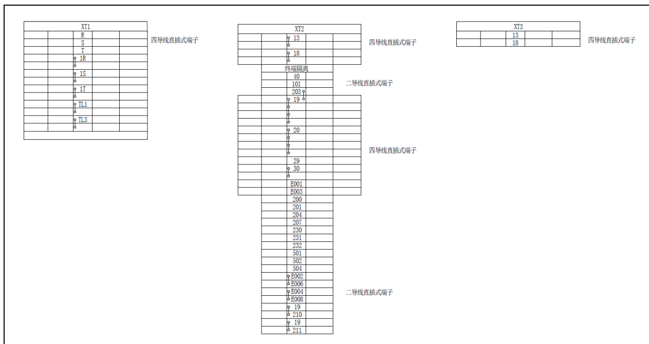
图 11.5 接线端子排接线图（ER6/12/20/30）
