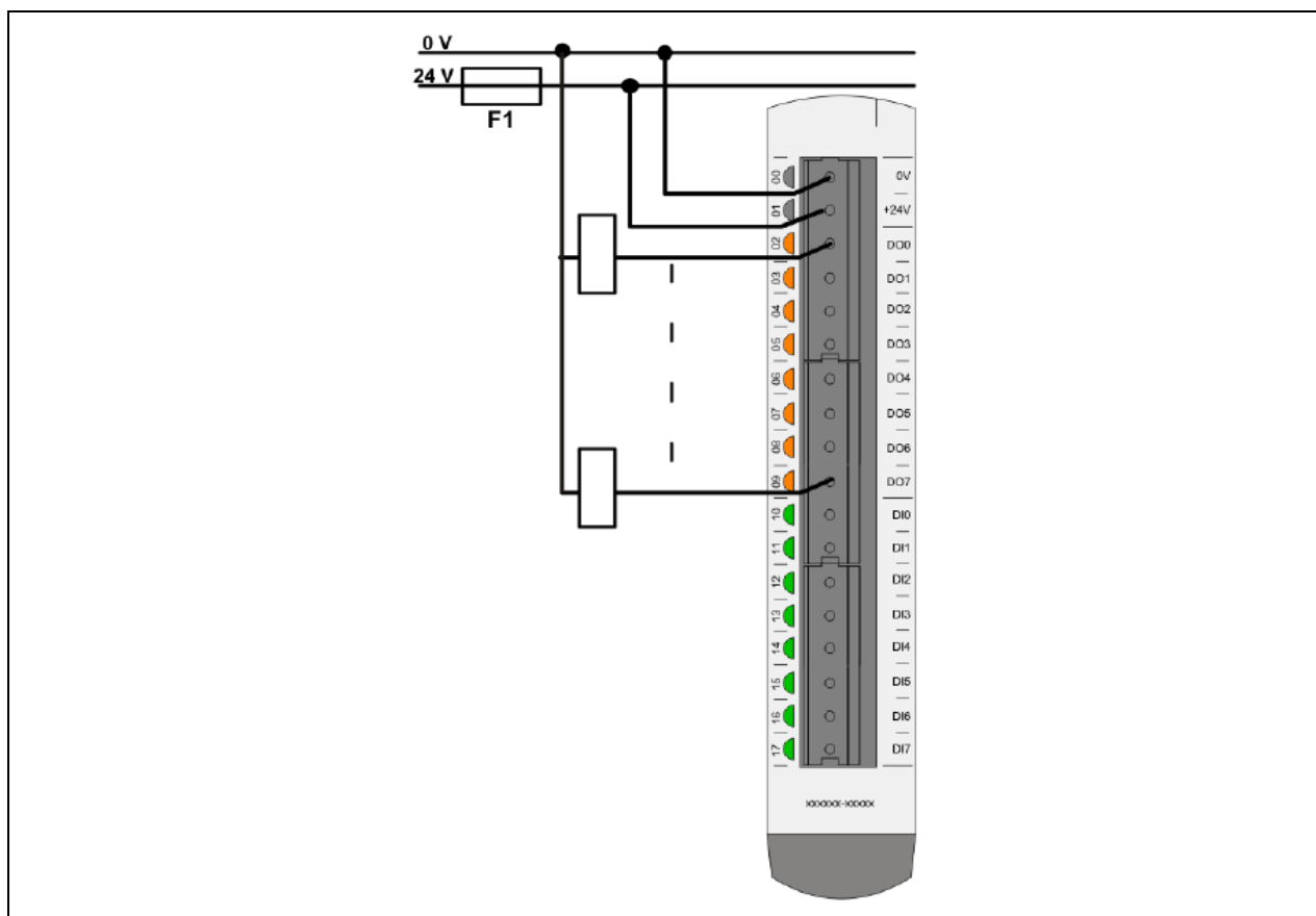
图 6.3 输出模块接线示意图
