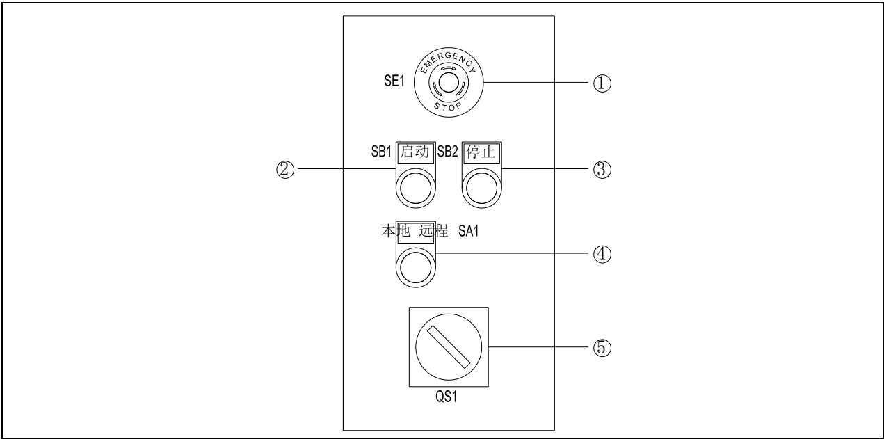
图 1.4 控制柜面板按钮示意图
