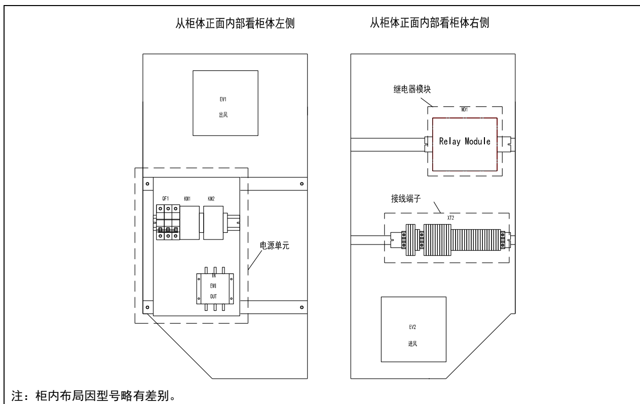
图 1.8 电柜内部布局（2）
