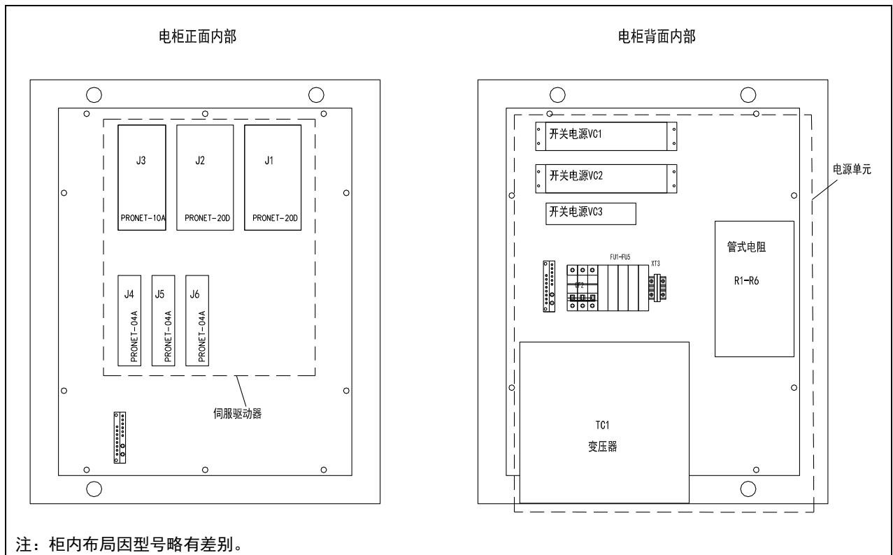
图 1.7 电柜内部布局（1）
