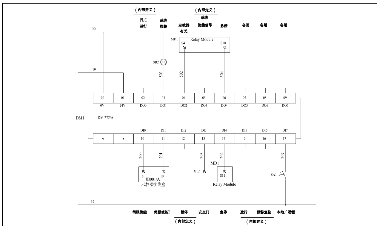
图 11.3 专用输入输出模块接线图
