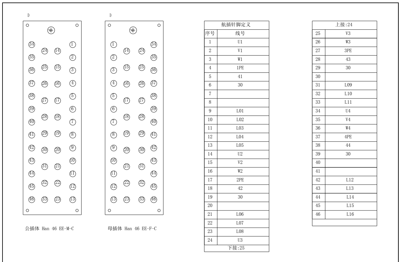
图 11.13 动力航插接线图 (ER180)
