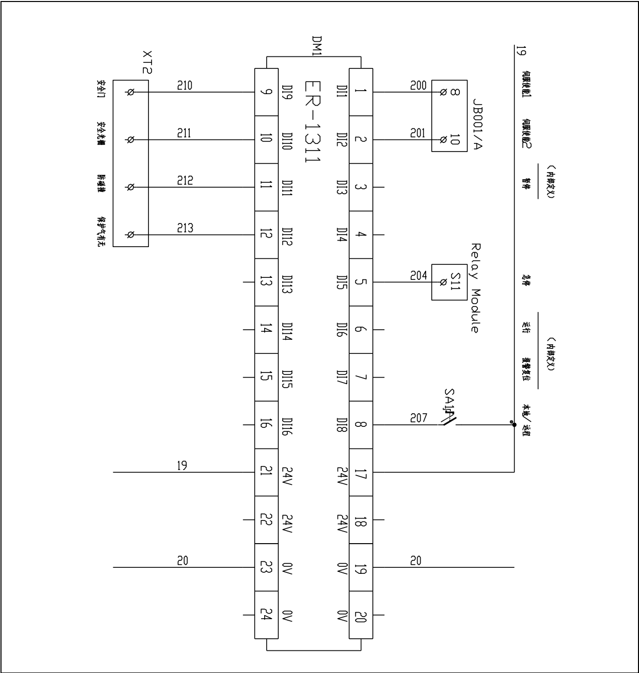
图 11.1 输入模块接线图
