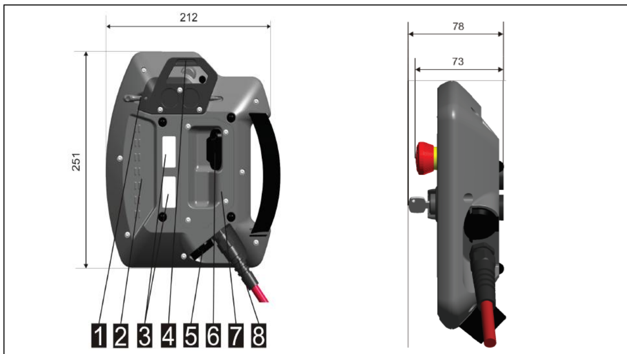
图 1.6 T70 示教器按钮示意图（背面、侧面）
