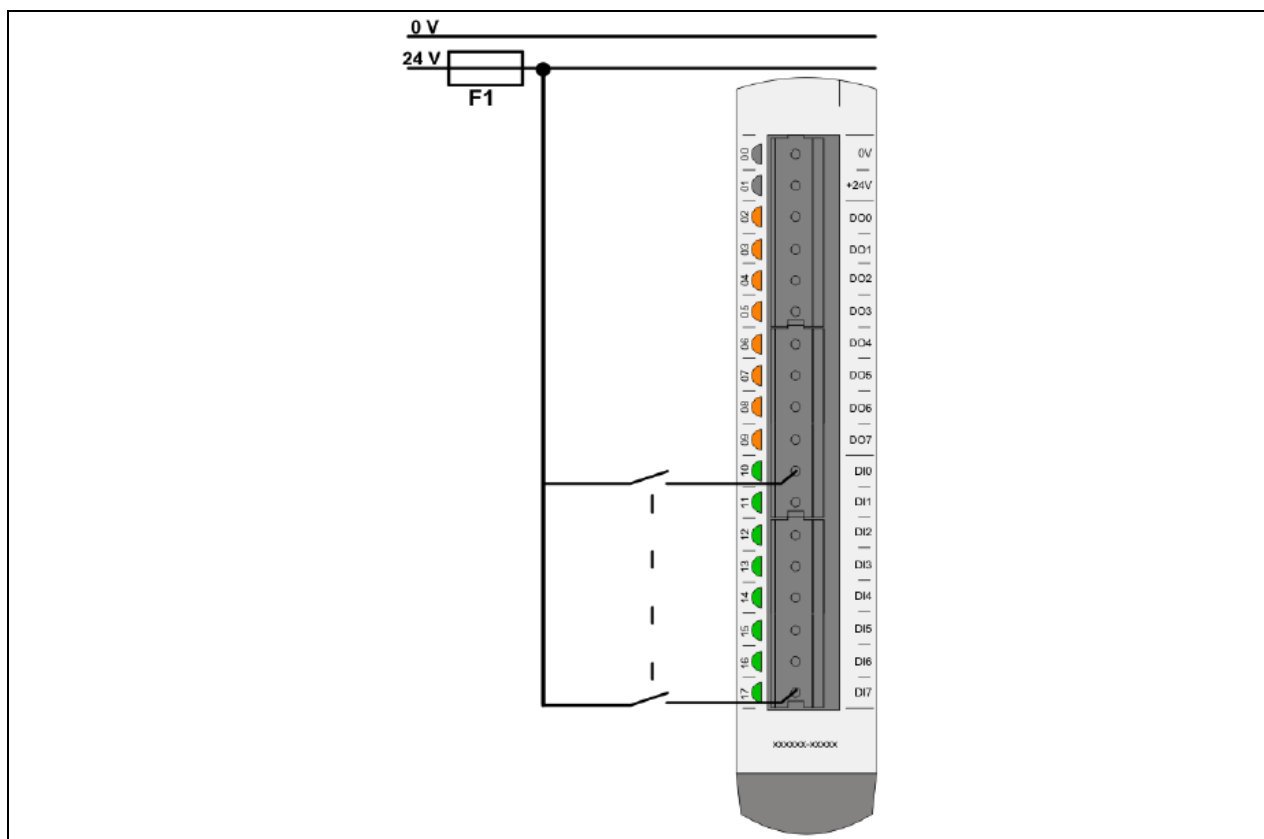
图 6.2 输入模块接线示意图
