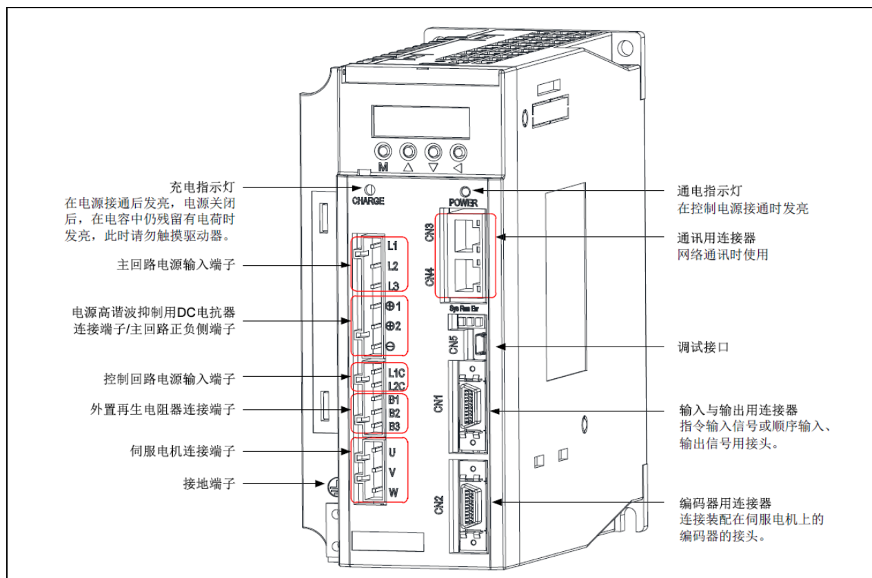
图 5.2 驱动器接线端口及功能分布
