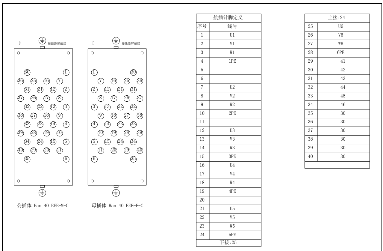
图 11.10 动力航插接线图 (ER6/30/80/120)
