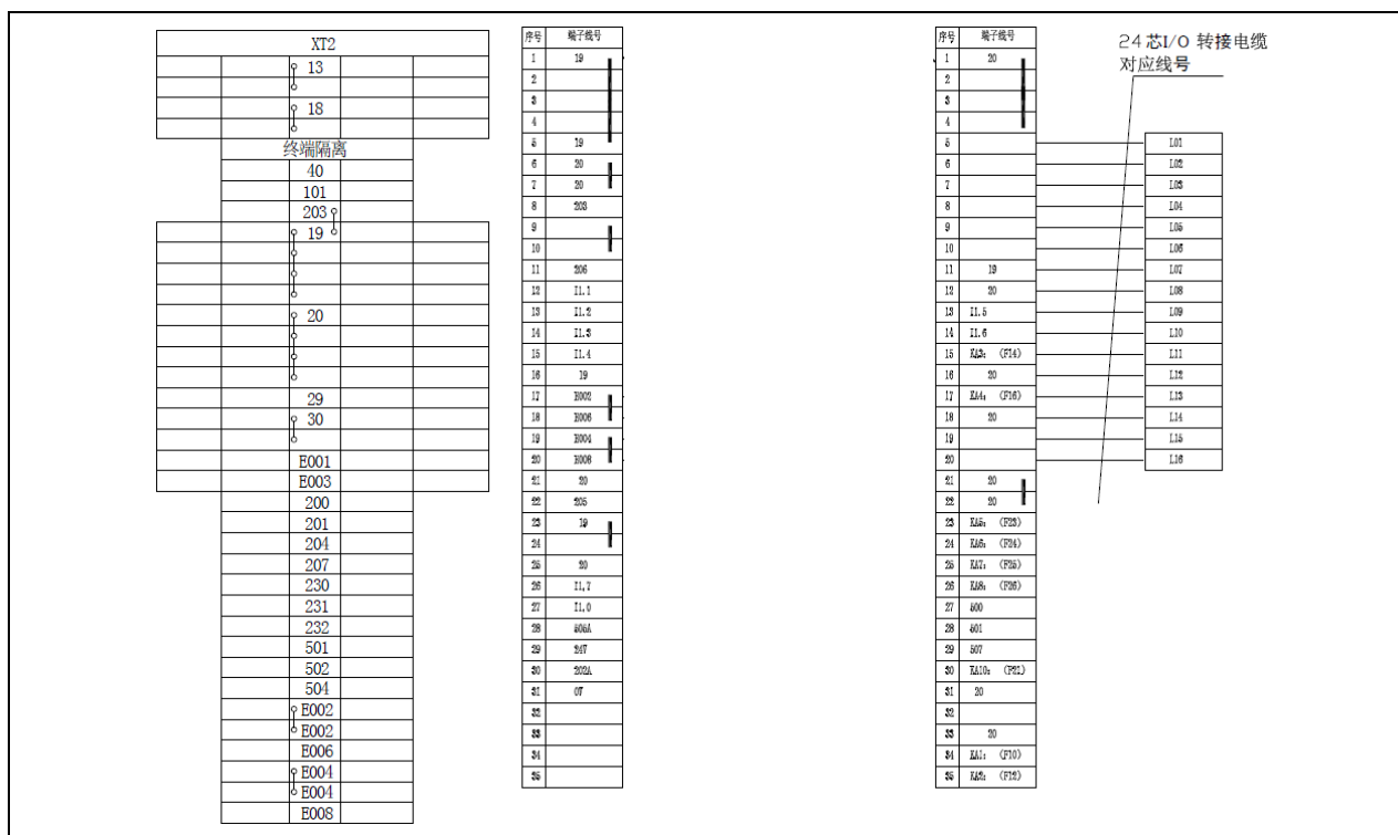
图 11.6 接线端子排接线图（ER80）
