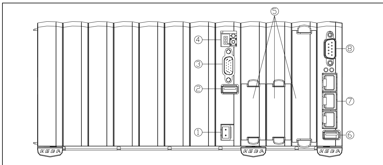
图 4.1 控制单元的接口布局（CP 控制器）
