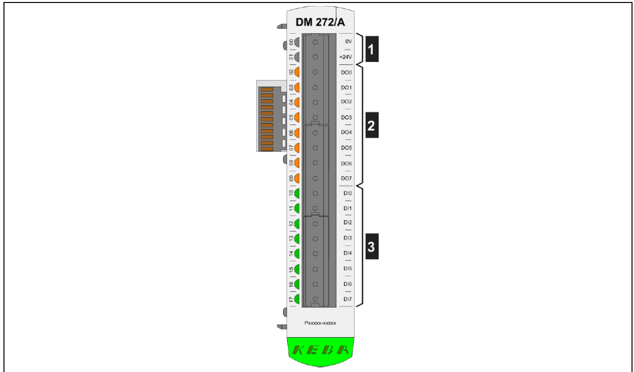
图 6.1 输入输出接口图示
