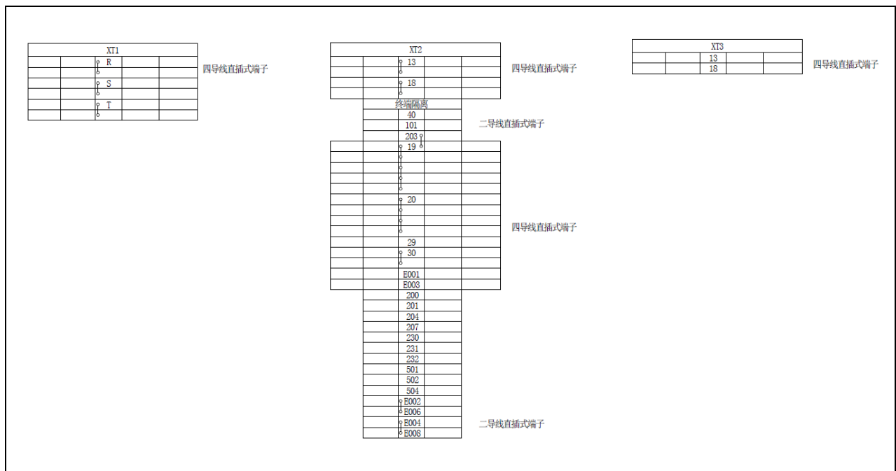
图 11.7 接线端子排接线图（ER180）
