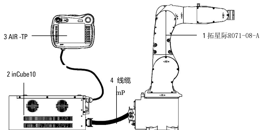
图 2-1 机器人系统的构成
