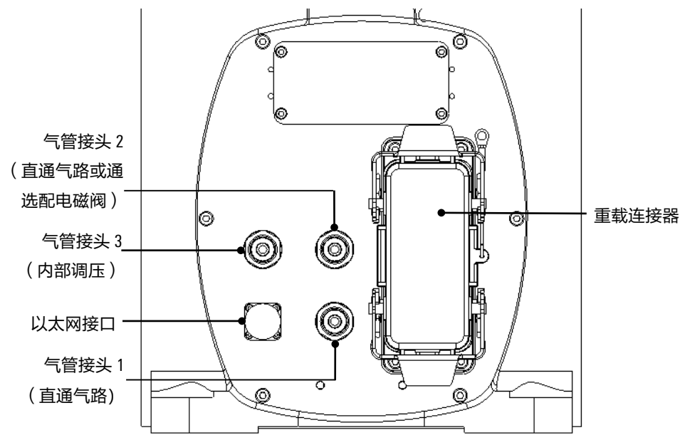
图 7-1 拓星际R071-08-A 型操作机本体上重载连接器
