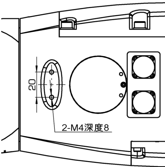
图 9-6 拓星际R071-08-A 型操作机小臂接口尺寸图
