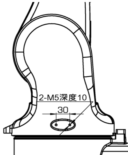
图 9-8 拓星际R071-08-A J1 轴本体接口尺寸图
