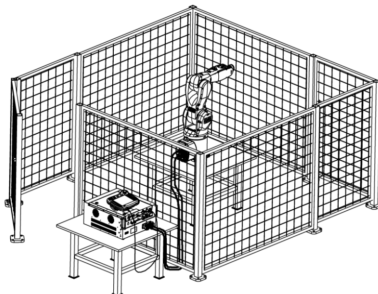
图 1 工业机器人安全工作示意图
