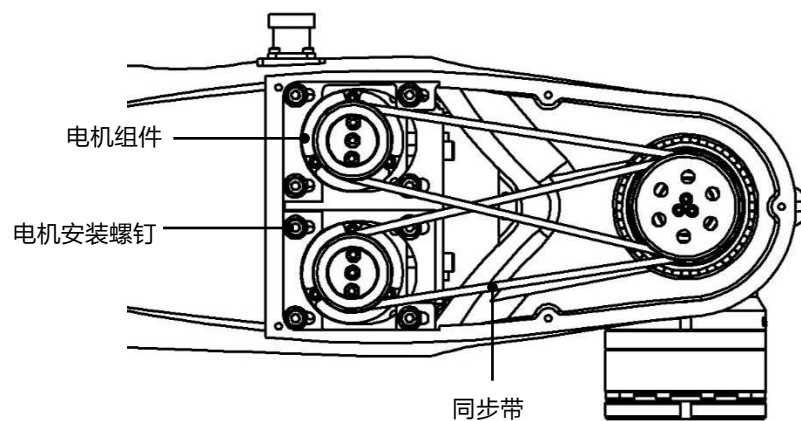
图 13-5 拆卸盖板
