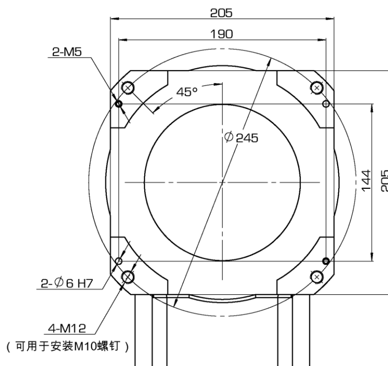
图 6-1 拓星际R071-08-A 型操作机基座接口尺寸
