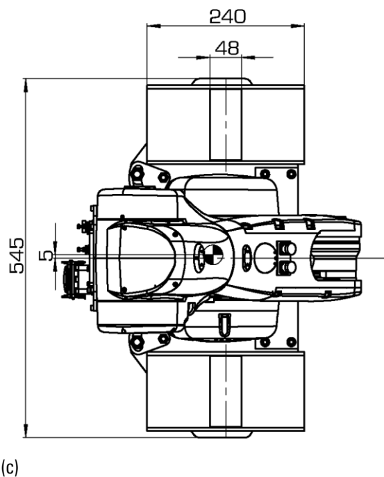
图 4-2 拓星际R071-08-A 搬运时 操作机尺寸
