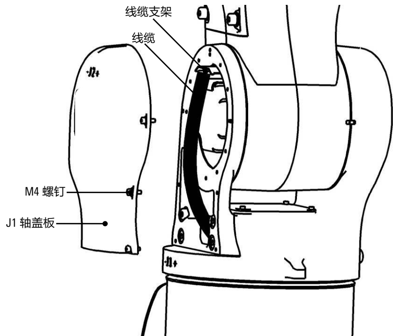
图 13-2 J1 轴本体内部线缆检修
