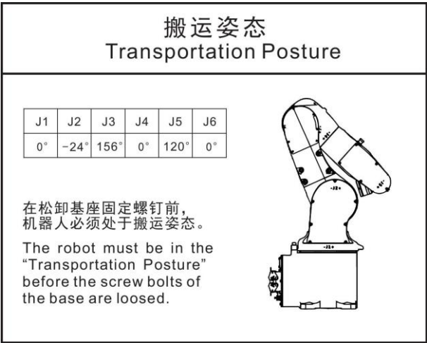
图 3-3 机器人搬运姿态标签
