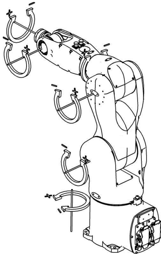
图 10-4 操作机各轴运动方向
