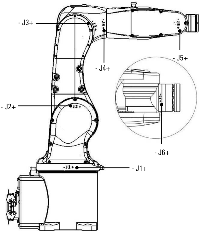
图 3-4 操作机上各轴方向标识
