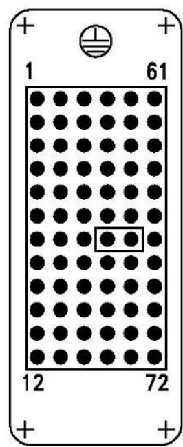
图 7-5 拓星际R071-08-A 型操作机重载接口
