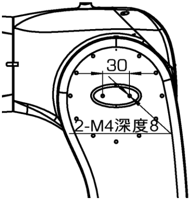
图 9-7 拓星际R071-08-A 大臂接口尺寸图
