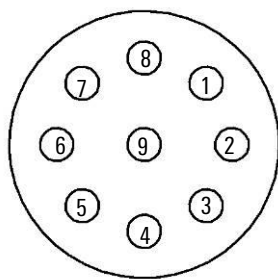
图 7-6 拓星际R071-08-A 型操作机用户 I0 接口
