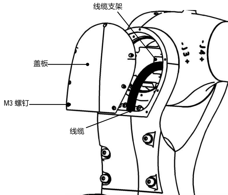
图 13-3 大臂内部线缆检修
