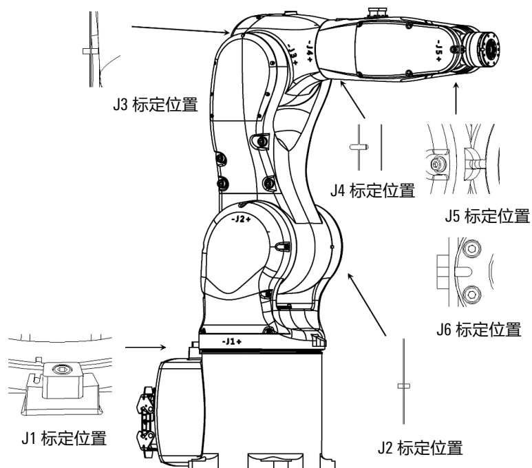
图 10-1 拓星际R071-08-A 型操作机各轴零点示意图
