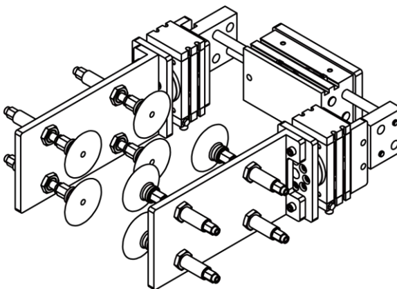
图 8-2 工业机器人用吸盘
