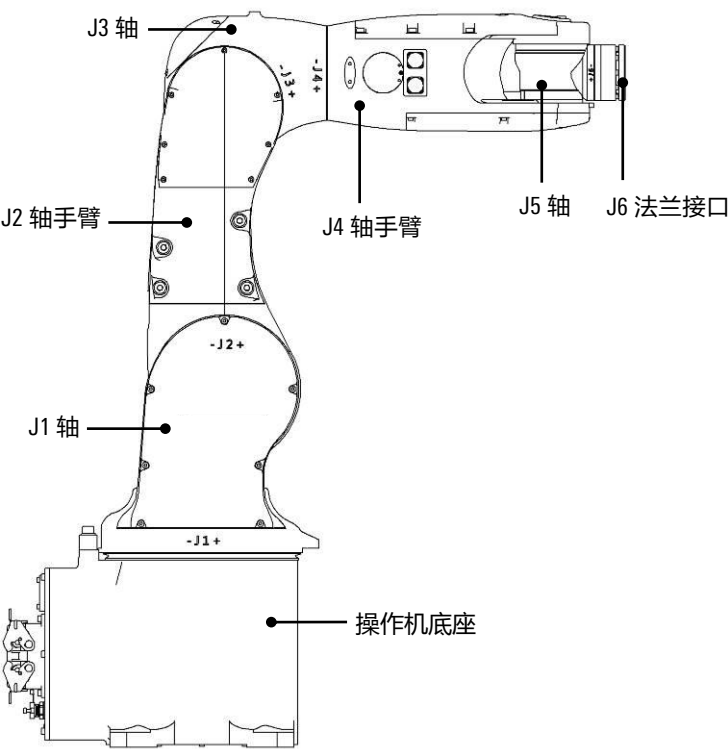
图 2-2 拓星际R071-08-A 型机器人本体及其各个部分
