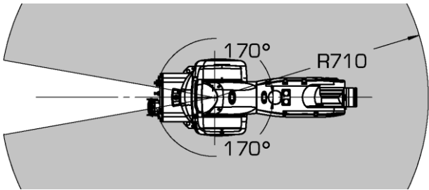
图 9-1 拓星际R071-08-A 型操作机工作范围
