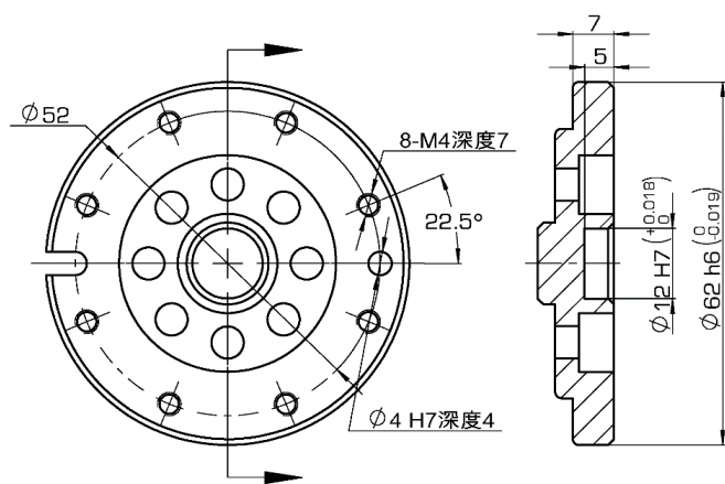
图 9-3 拓星际R071-08-A 型操作机腕部法兰尺寸示意图
