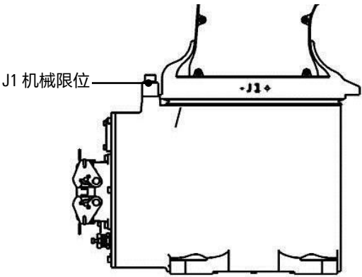
图 9-2 拓星际R071-08-A 型操作机上机械式制动器
