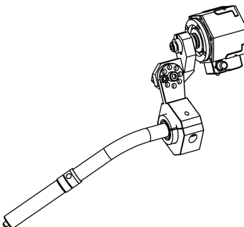
图 8-3 工业机器人用弧焊枪
