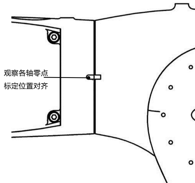
图 10-2 肉眼观察零点标定方式
